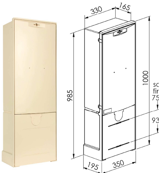
Dimensions REMBT 300
